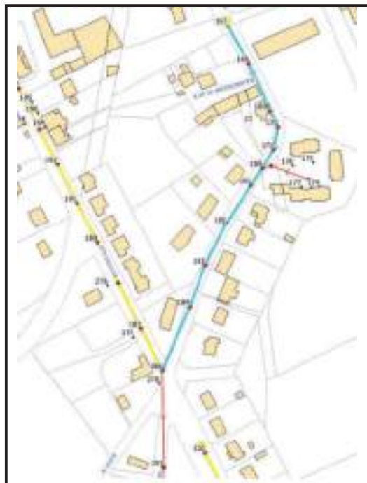
Plan de situation des tronçons à réhabiliter rue du Lac aux Fées
